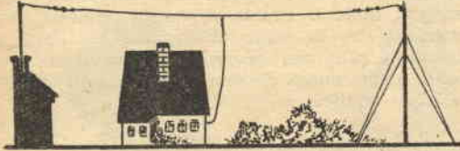
Antenna semplice a «T».
